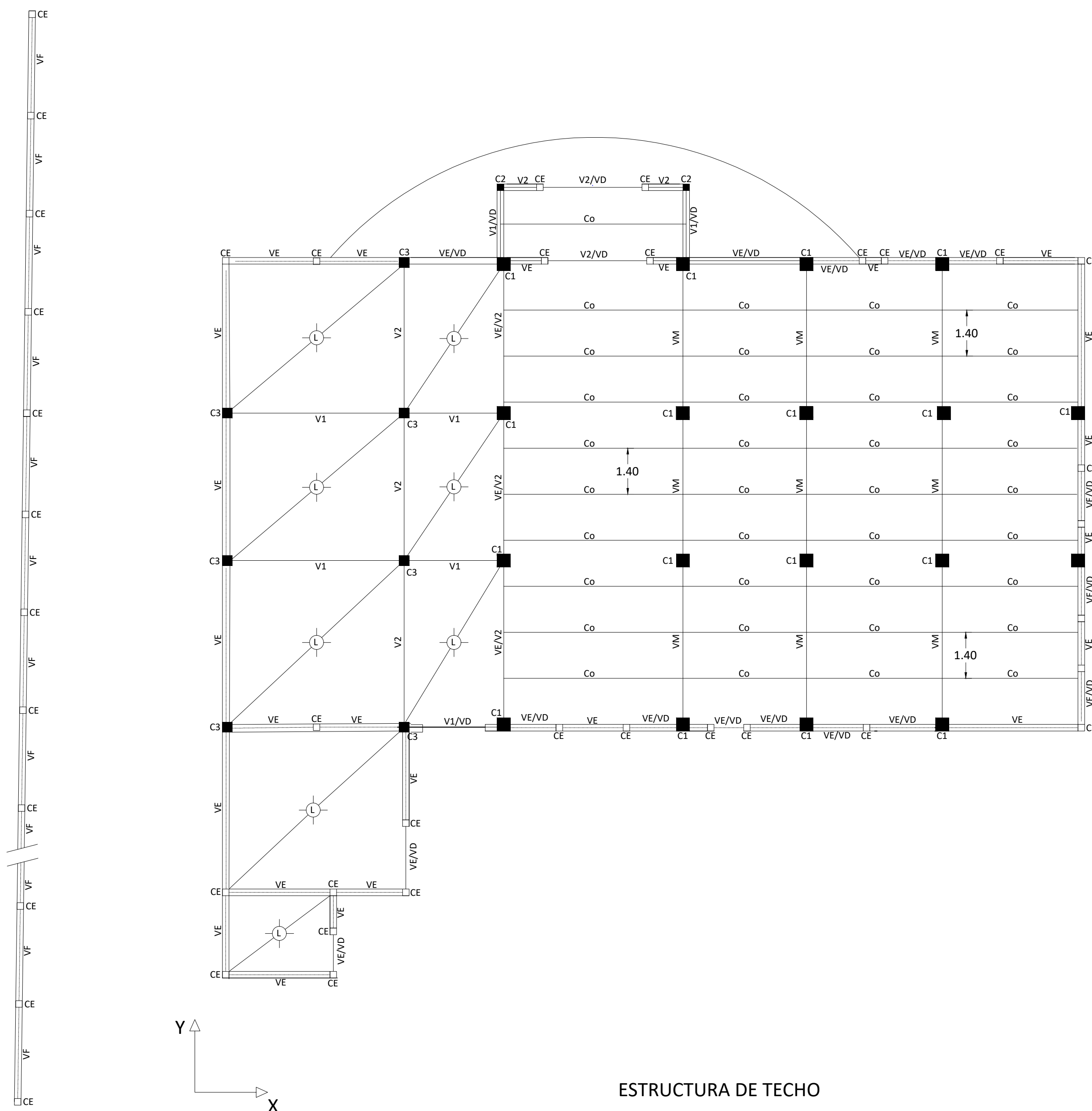
ESTRUCTURA DE TECHO
