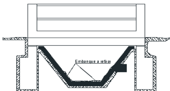
PUENTE SOBRE CANAL / RAMO IMPERMEABILIZADO SECCIÓN TRAPEZOIDAL
