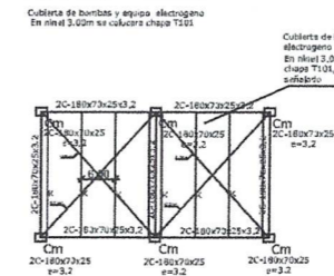
NIVEL +3.00
