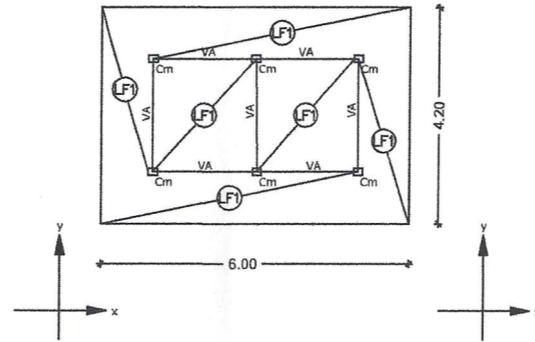
FUNDACIONES
