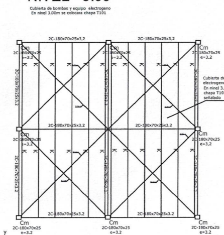
NIVEL +3.00
