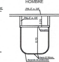
DETALLE GUARDA HOMBRE
