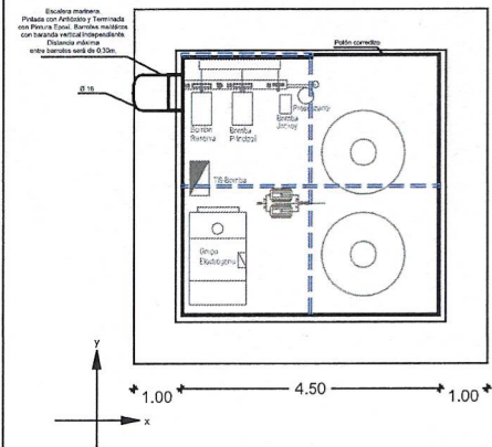
ESQUEMA ESTRUCTURAL TIPO
