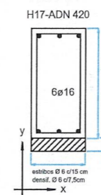
Detalle Piso de Tanques
