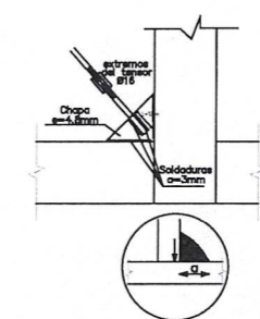
Detalle Piso de Tanques
