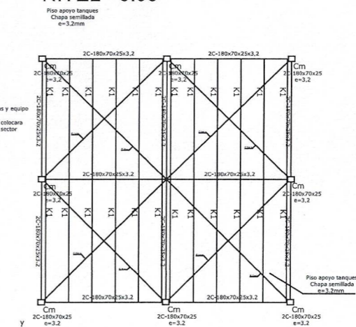
NIVEL +6.00
