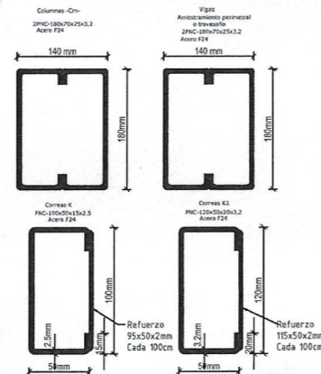
SECCIONES DE VIGAS Y COLUMNAS
